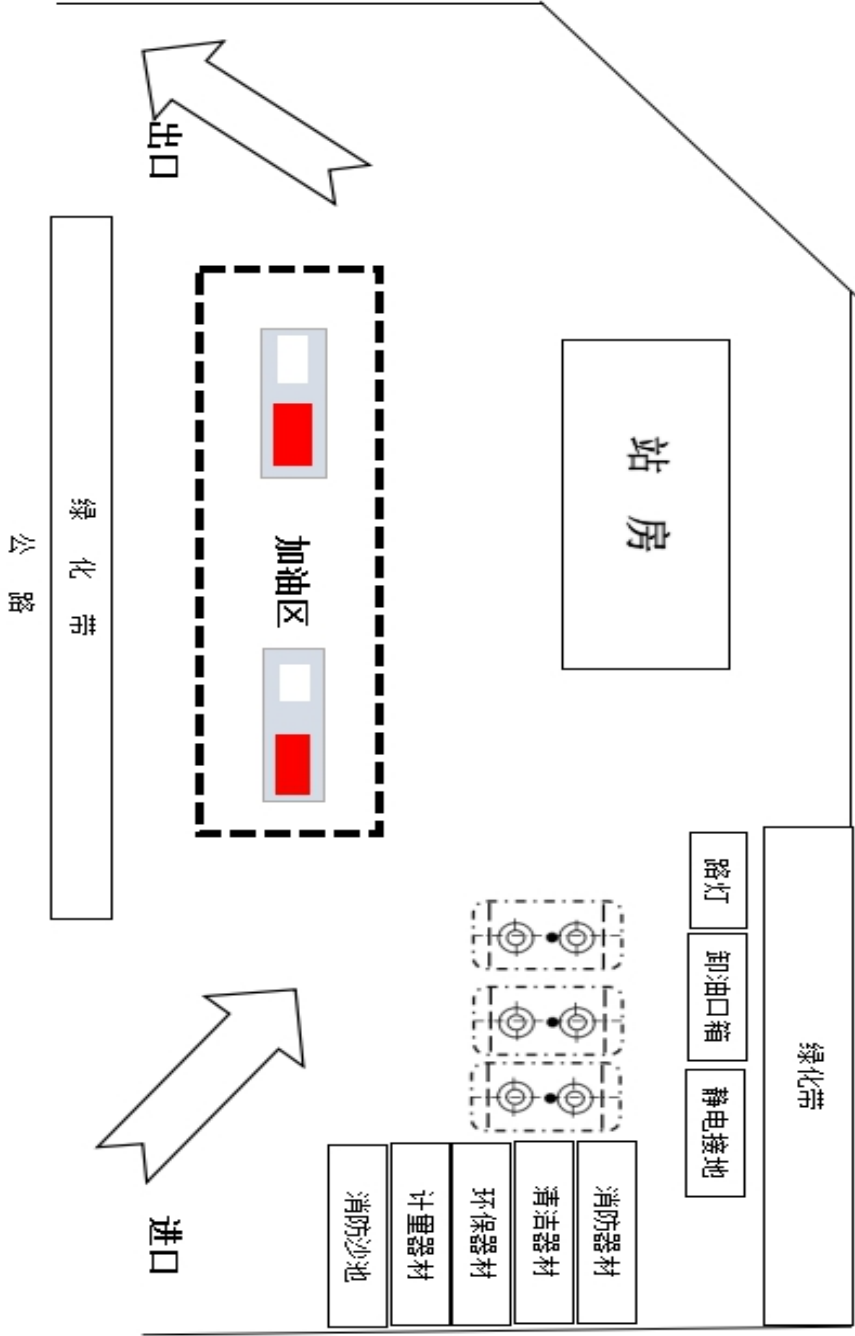
附件 5 总平面布置图
