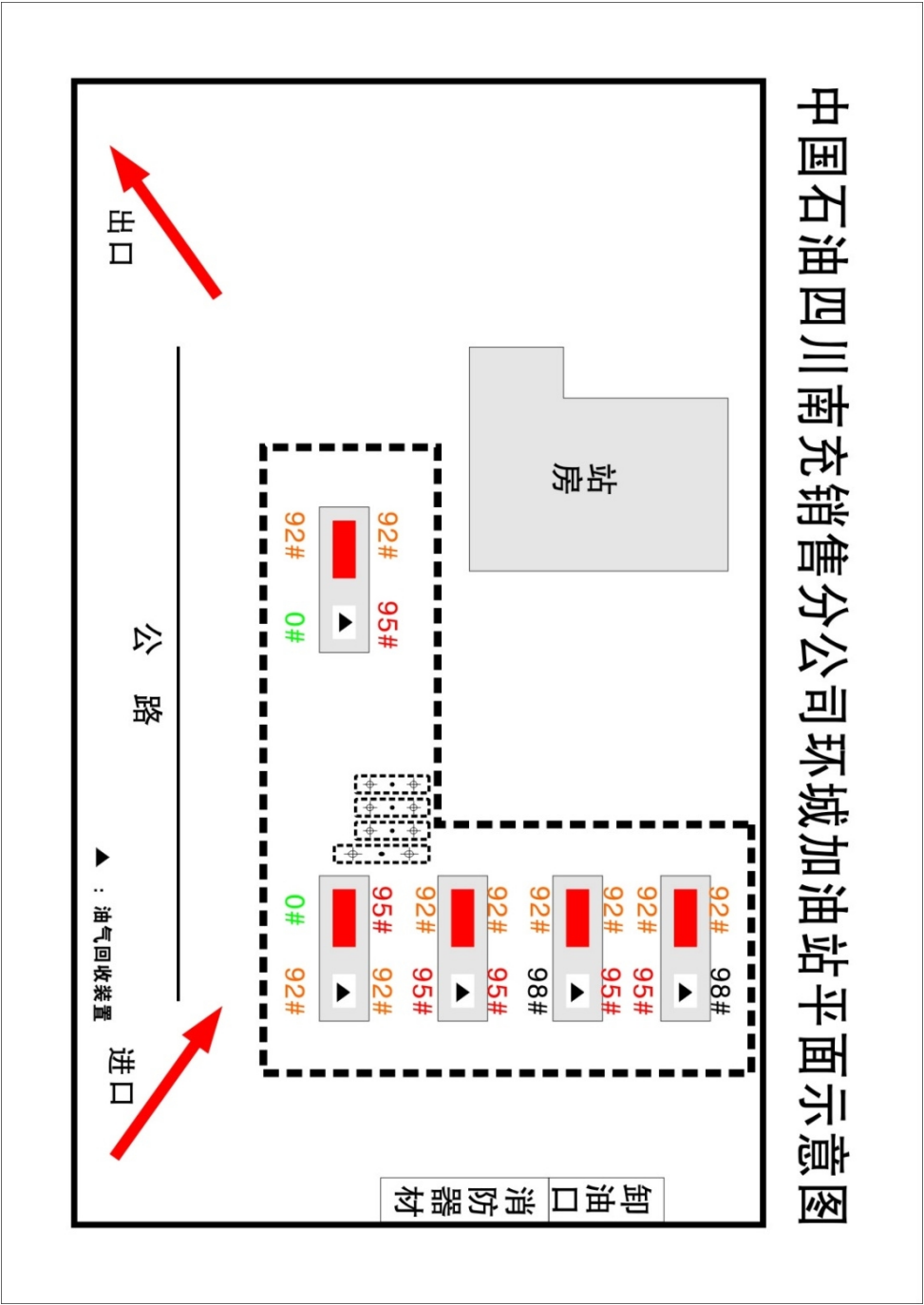
附件 5 总平面布置图
