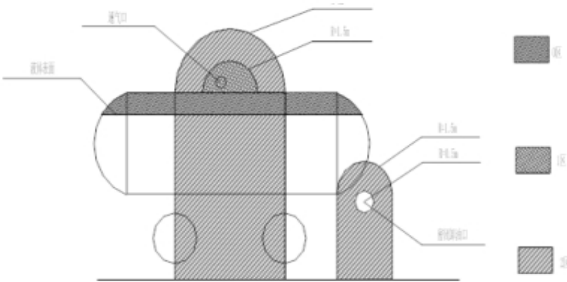
图 3-2 油罐车卸油爆炸危险区域划分
