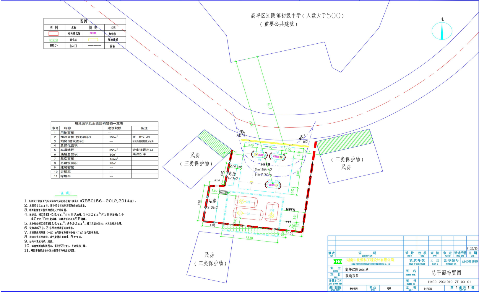
附件 9 加油站总平面布置图
