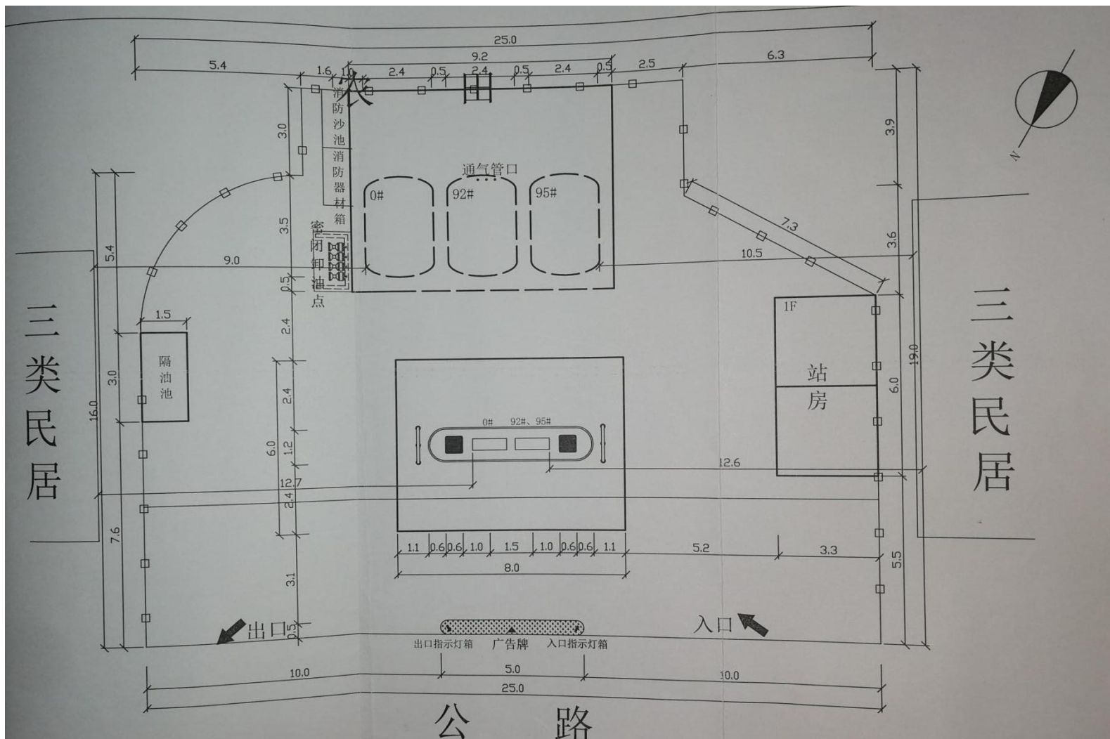
附件 5 加油站总平面设计图
