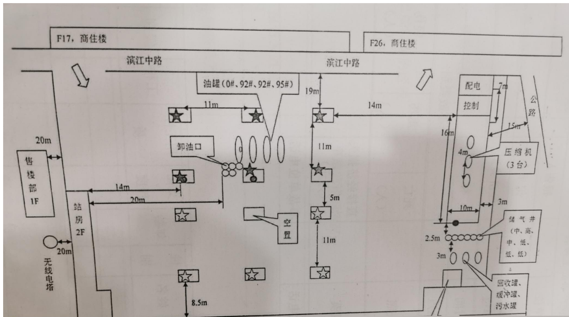
附件 5 加油加气站总平面布置图
