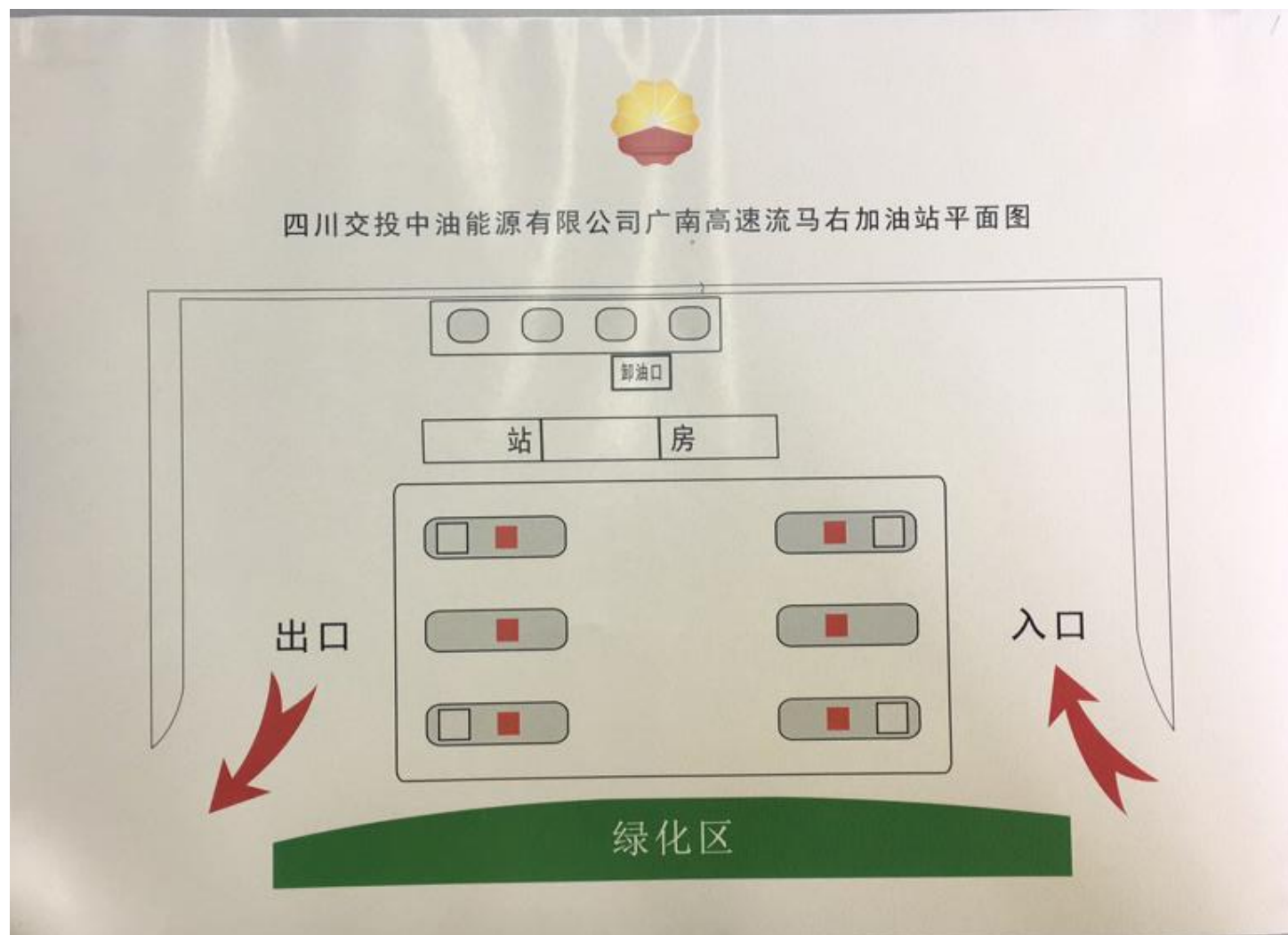
附件 5 加油站总平面设计图
