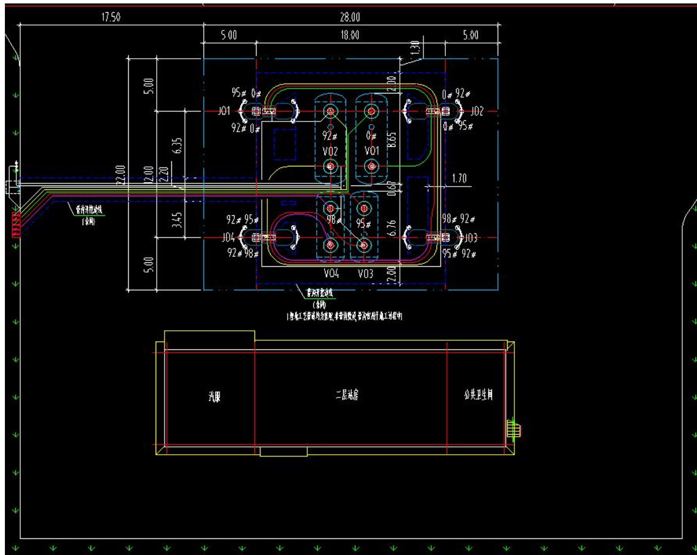
附件 5 加油站总平面设计图
