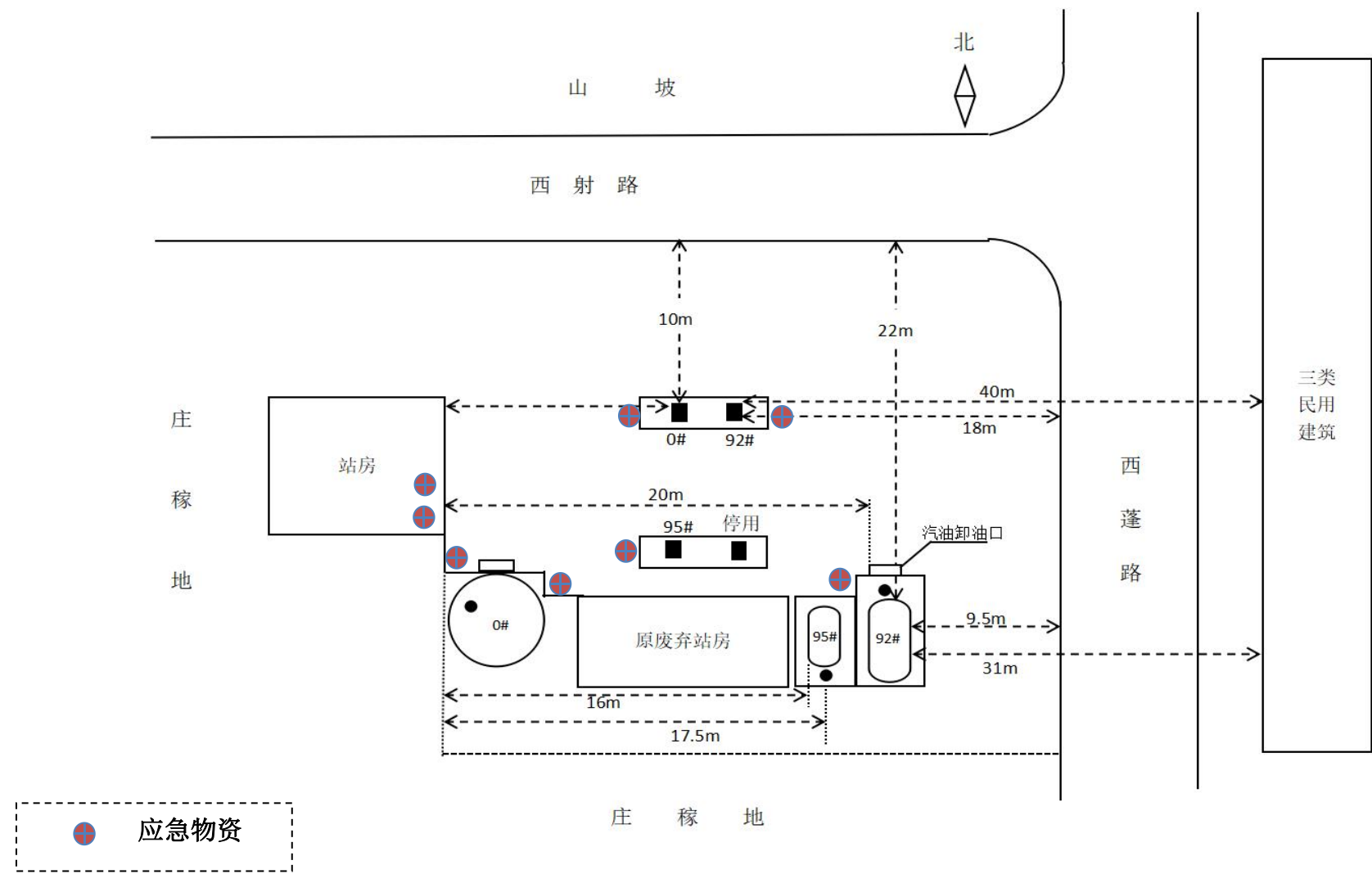
3、西充双凤仪垭加油站应急物资布置图
