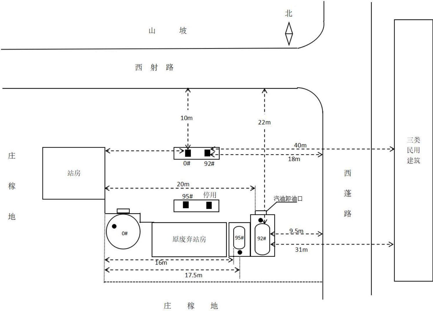
2、西充双凤仪垭加油站总平面布置图
