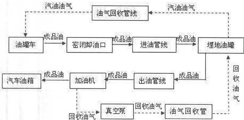
图2-4 加油站工艺流程图
