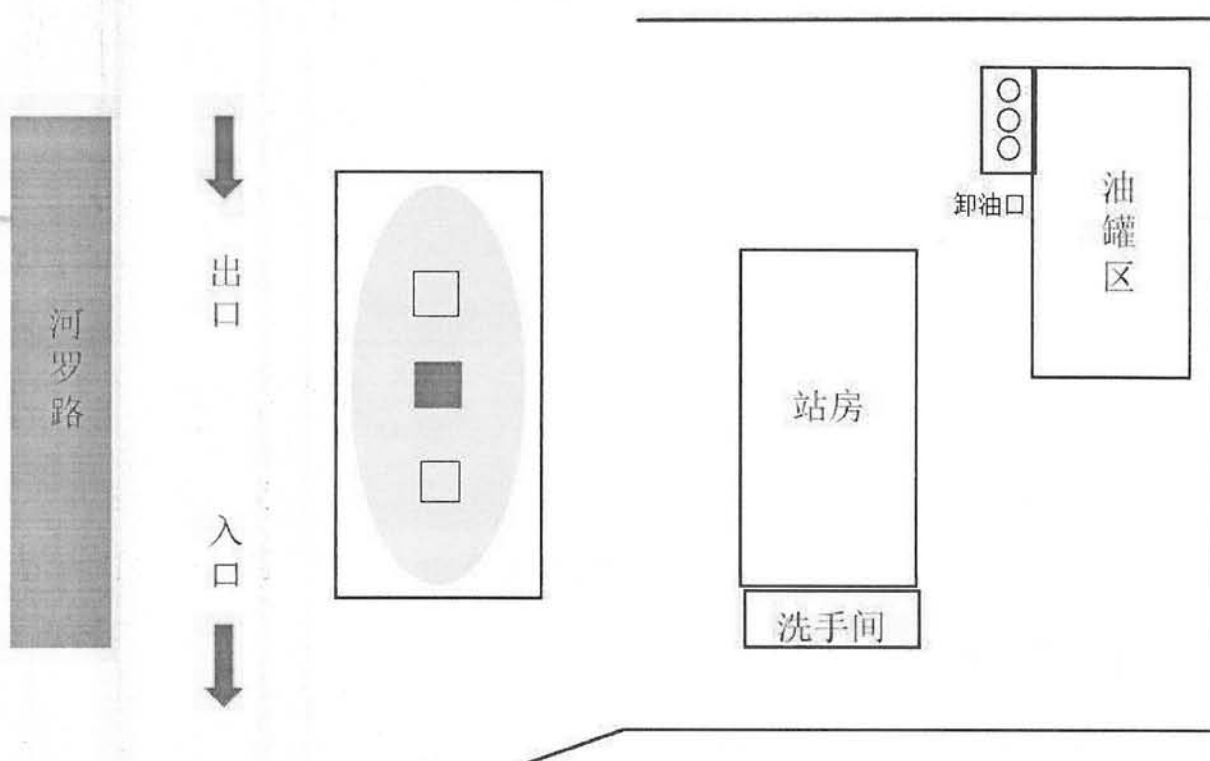
图 2-2 加油站总平面布置示意图
