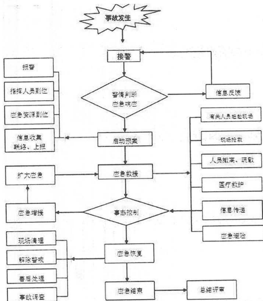
图 5-1 一级应急响应程序图
