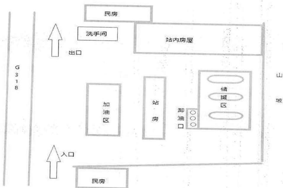
图 2-2 加油站总平面布置示意图
