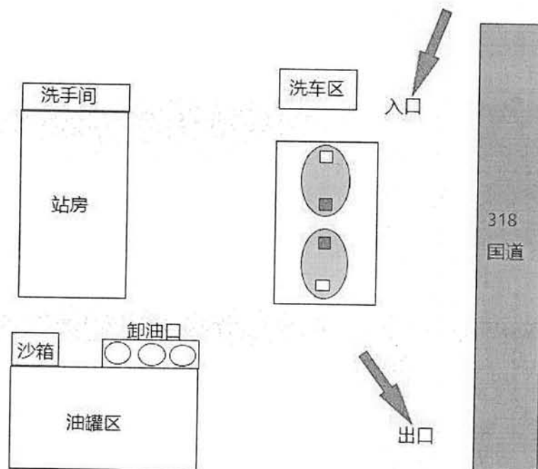
图 2-2 加油站总平面布置示意图
