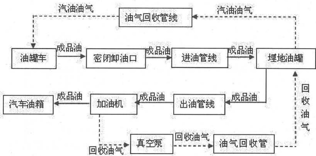
图2-4 加油站工艺流程图
