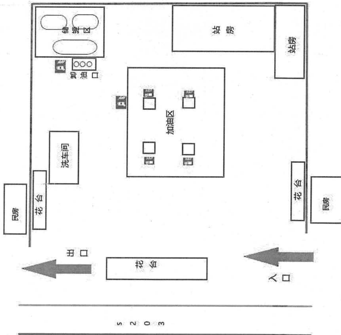
附件 8 消防器材布置示意图
