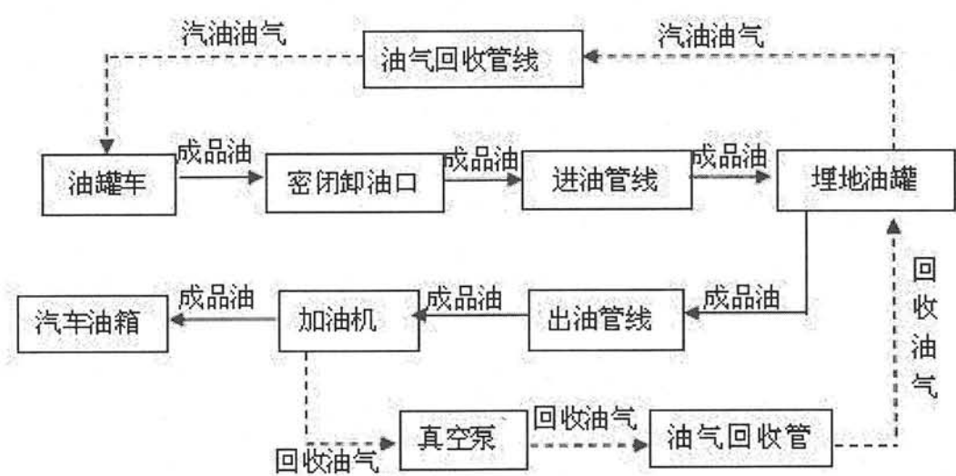
图2-4 加油站工艺流程图
