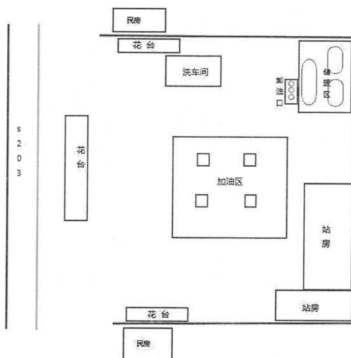
图 2-2 加油站总平面布置示意图
