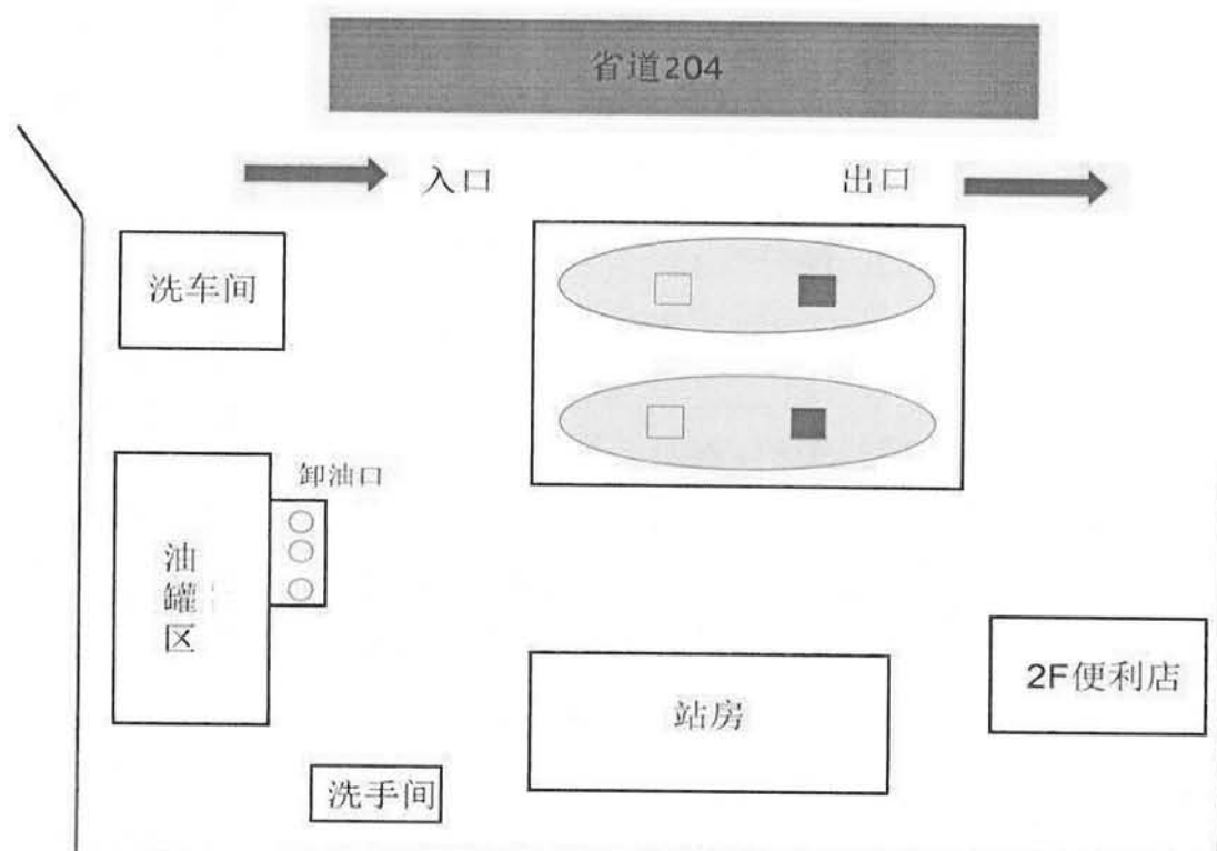
图 2-2 加油站总平面布置示意图
