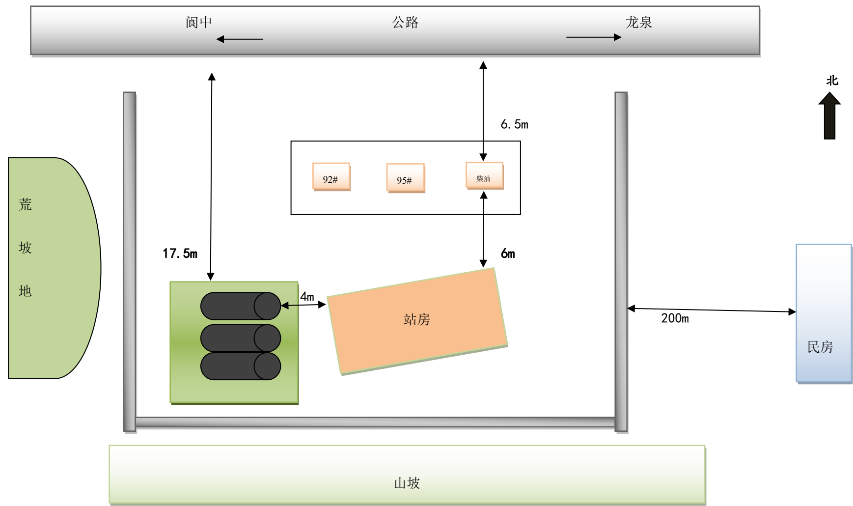
2、阆中市龙泉加油站总平面布置图
